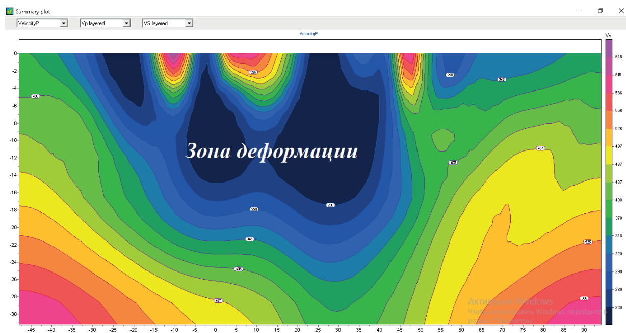
Рисунок 6. Зона распространения грунтов, которая может деформироваться
