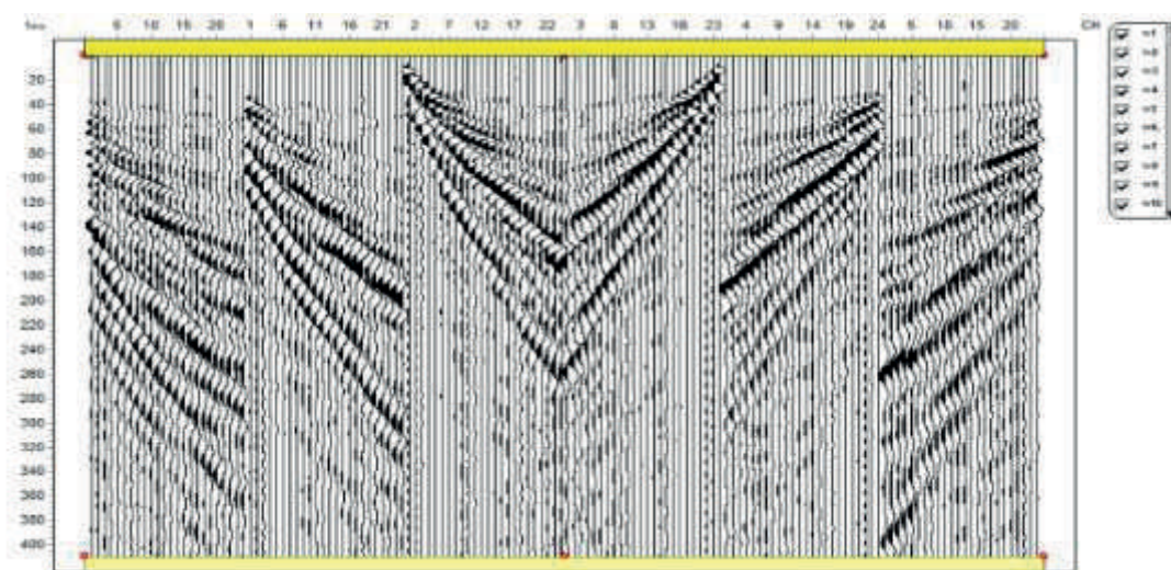
Рисунок 3. Регистрация поверхностных волн.
