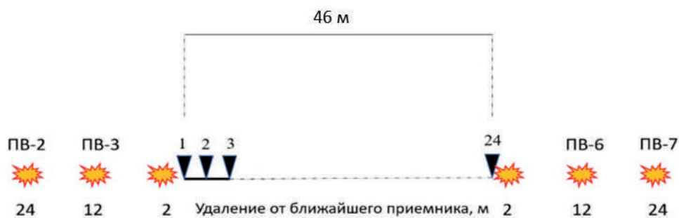
Рисунок 2. Схема производства сейсморазведочных работ MASW.
