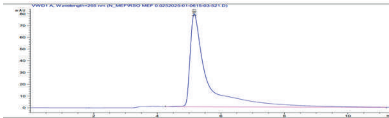
1-расм. Мефедроннинг ишчи стандарт эритмаси хроматограммаси
