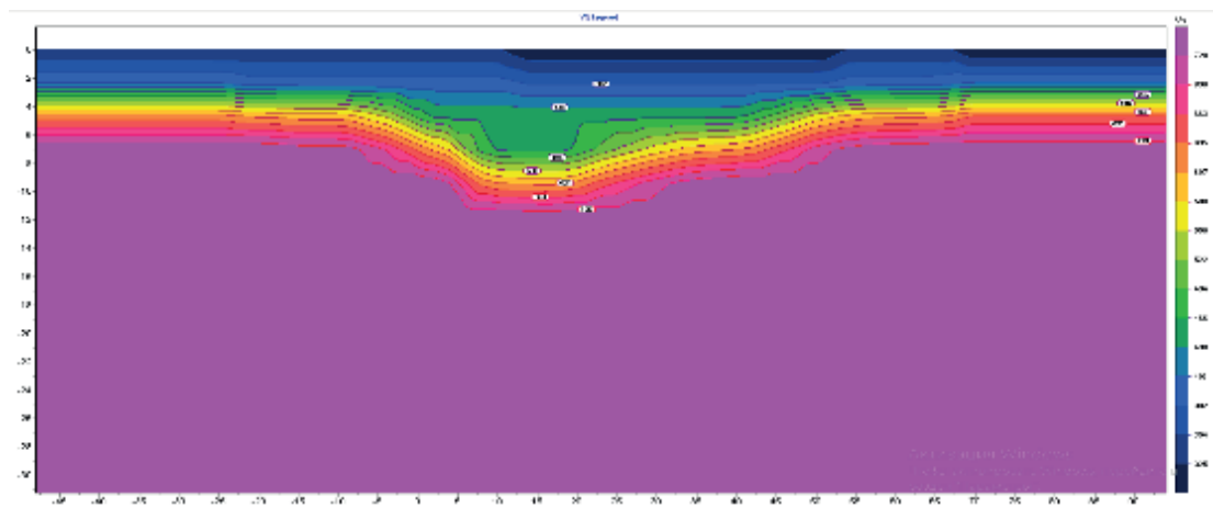
Рисунок 5. Слойные строения грунтов по параметру V_s
