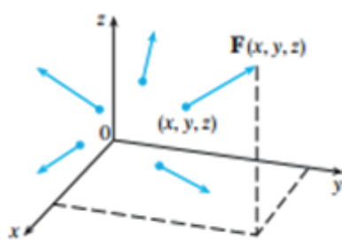
2-rasm. \mathbb{R}^3 dagi vektor maydon
