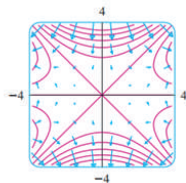
7-rasm. f(x, y) = x^2y - y^3 funksiya kontur kartasi bilan gradiyentning vektor maydoni grafigi
