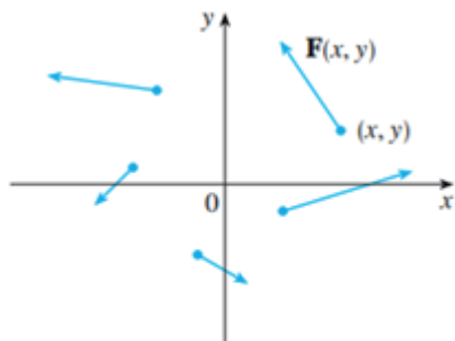
1-rasm. \mathbb{R}^2 dagi vektor maydon
