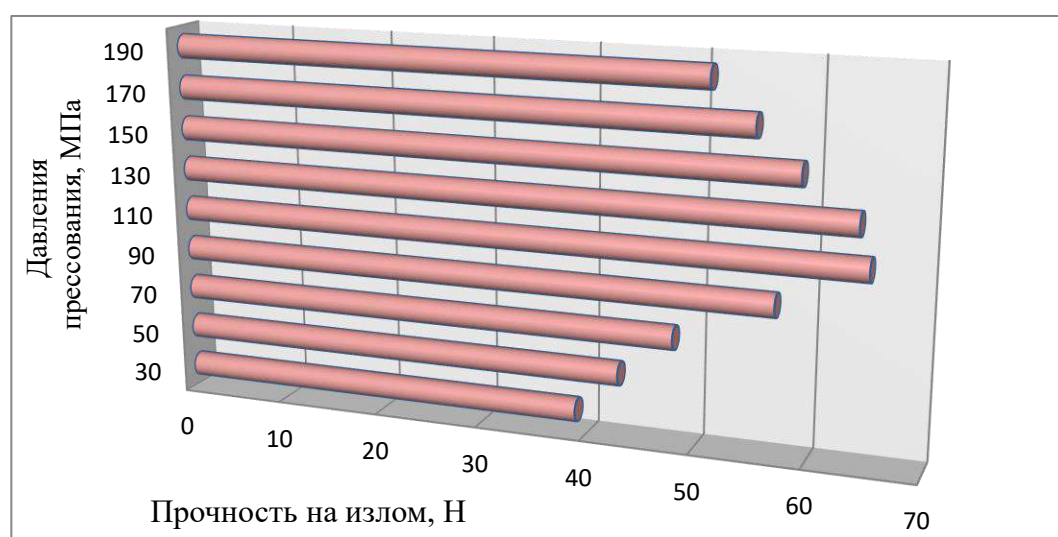
Рис. 1. Влияние давления прессования на устойчивость таблеток «Винамир» к раздавливанию
