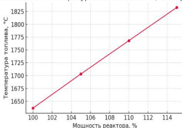
Рисунок 1– Зависимость максимальной температуры топлива от мощности реактора
