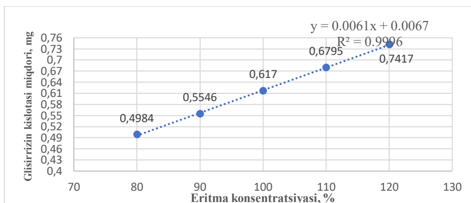
1-rasm. Uslubning chiziqliligini tekshirish uchun chizilgan grafik ( y=a \cdot x+b , a=0,0061 , b=0,0067 )
